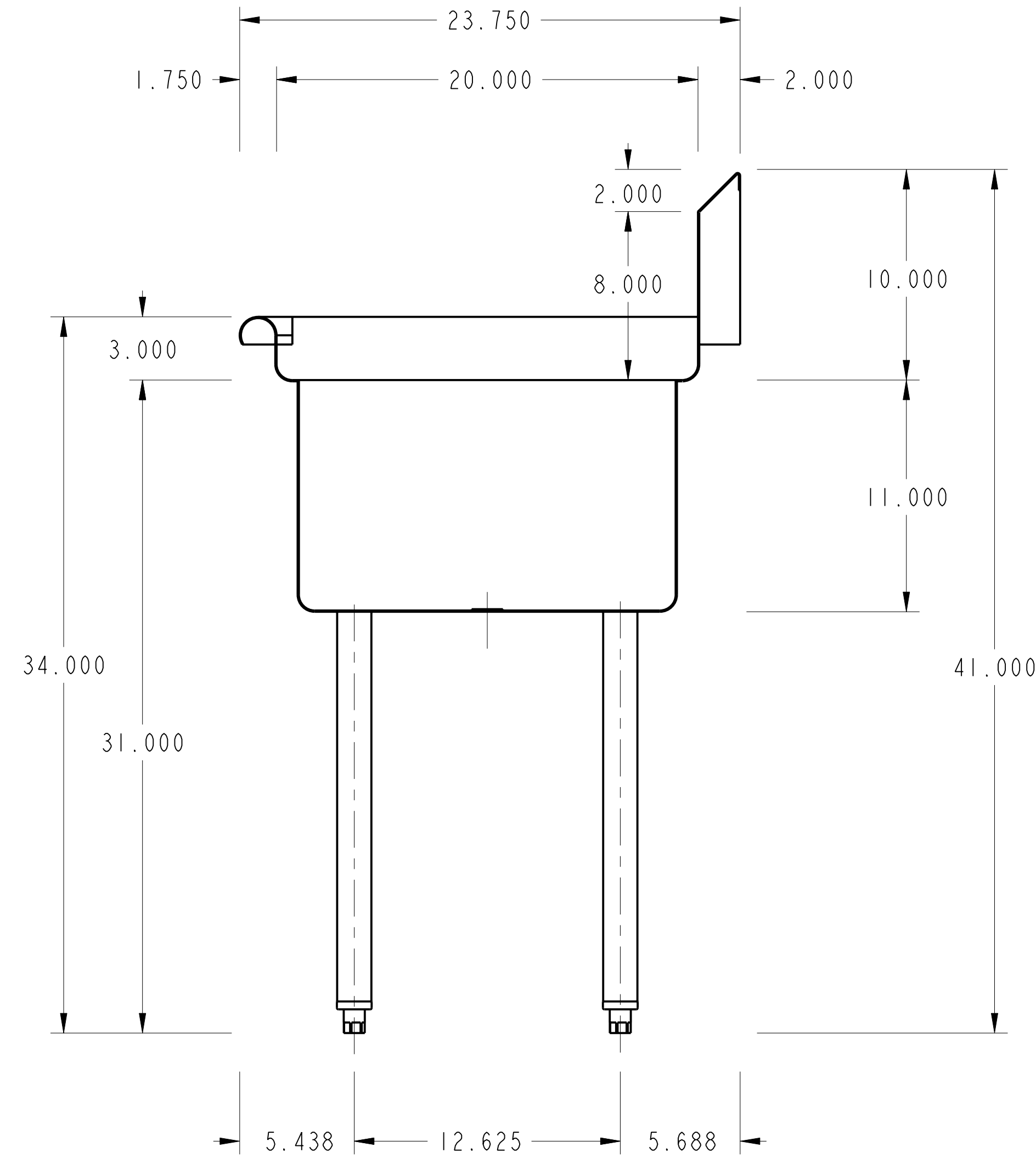
SECTION A-A
