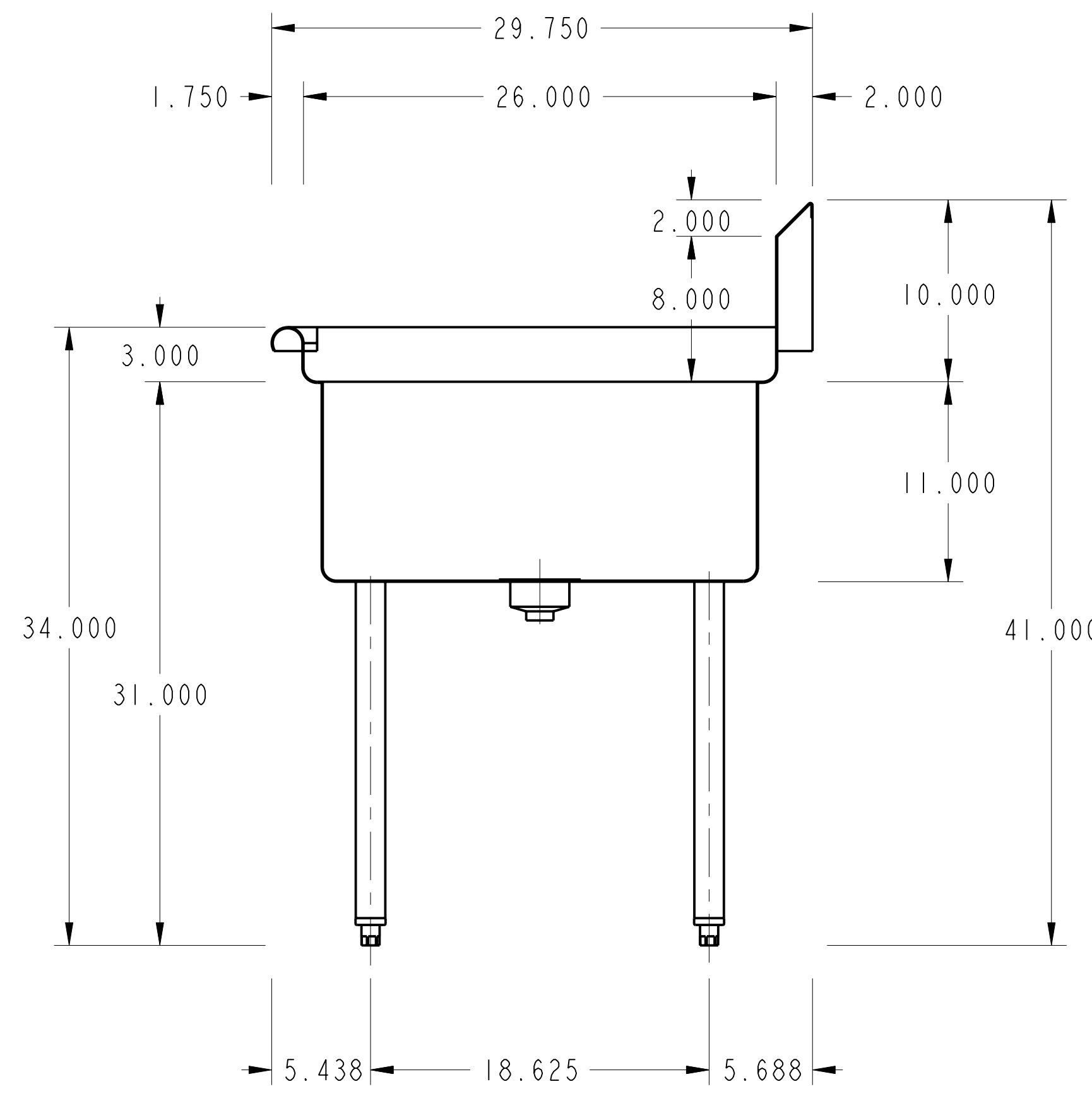
SECTION A-A
