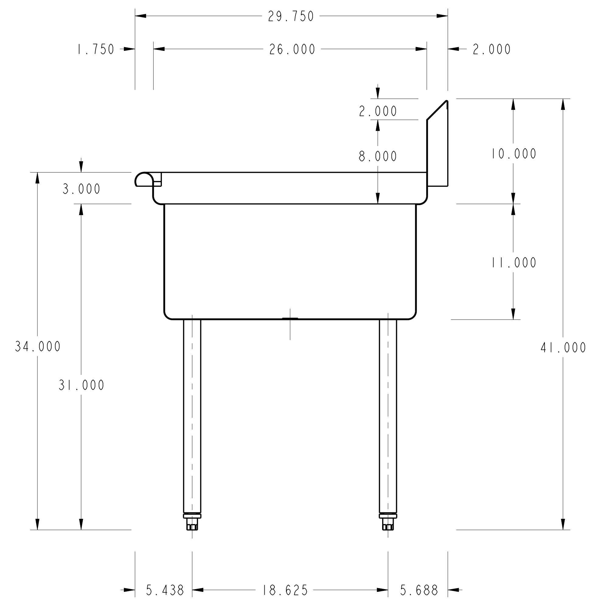
SECTION A-A
