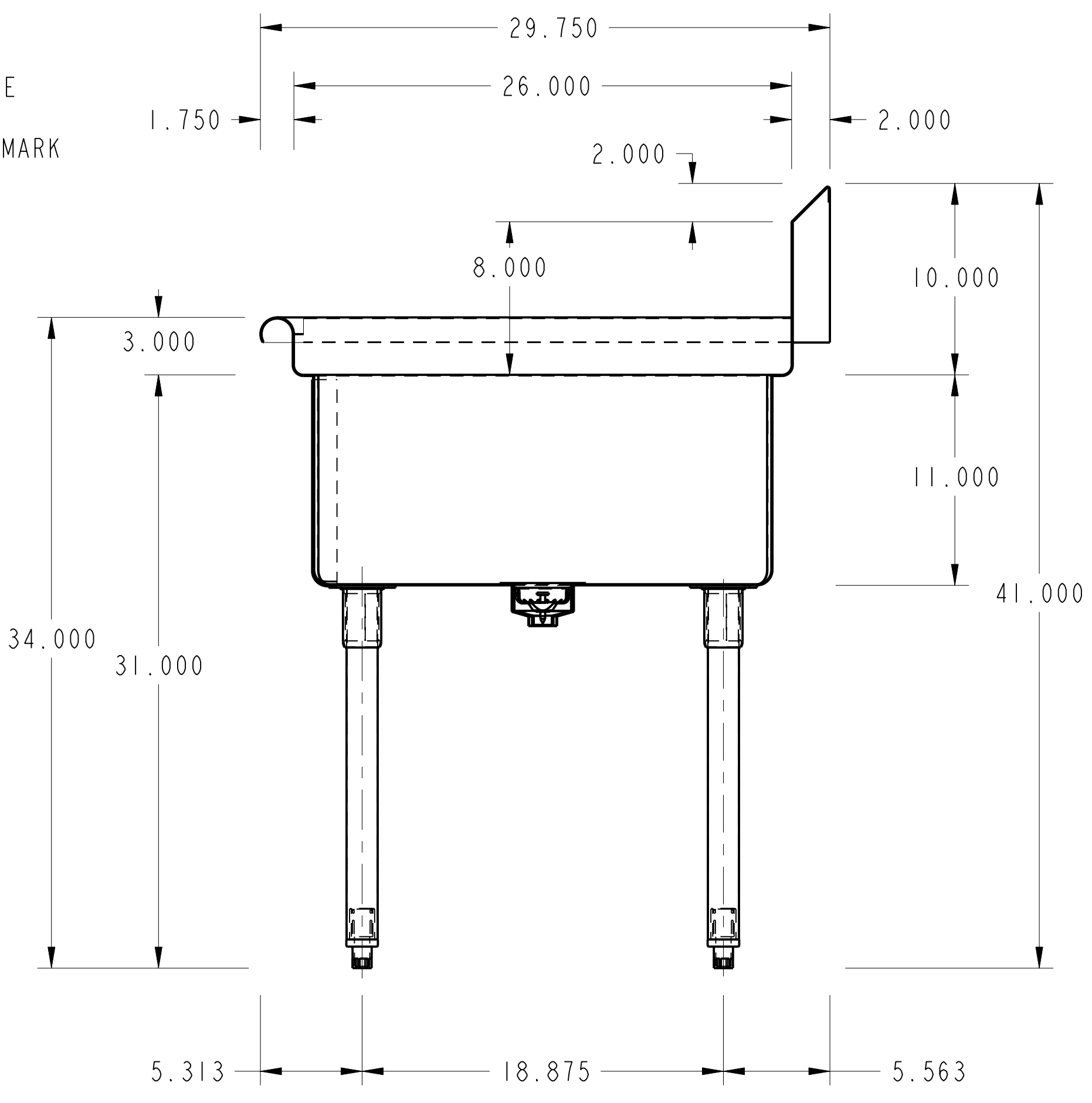
SECTION A-A
