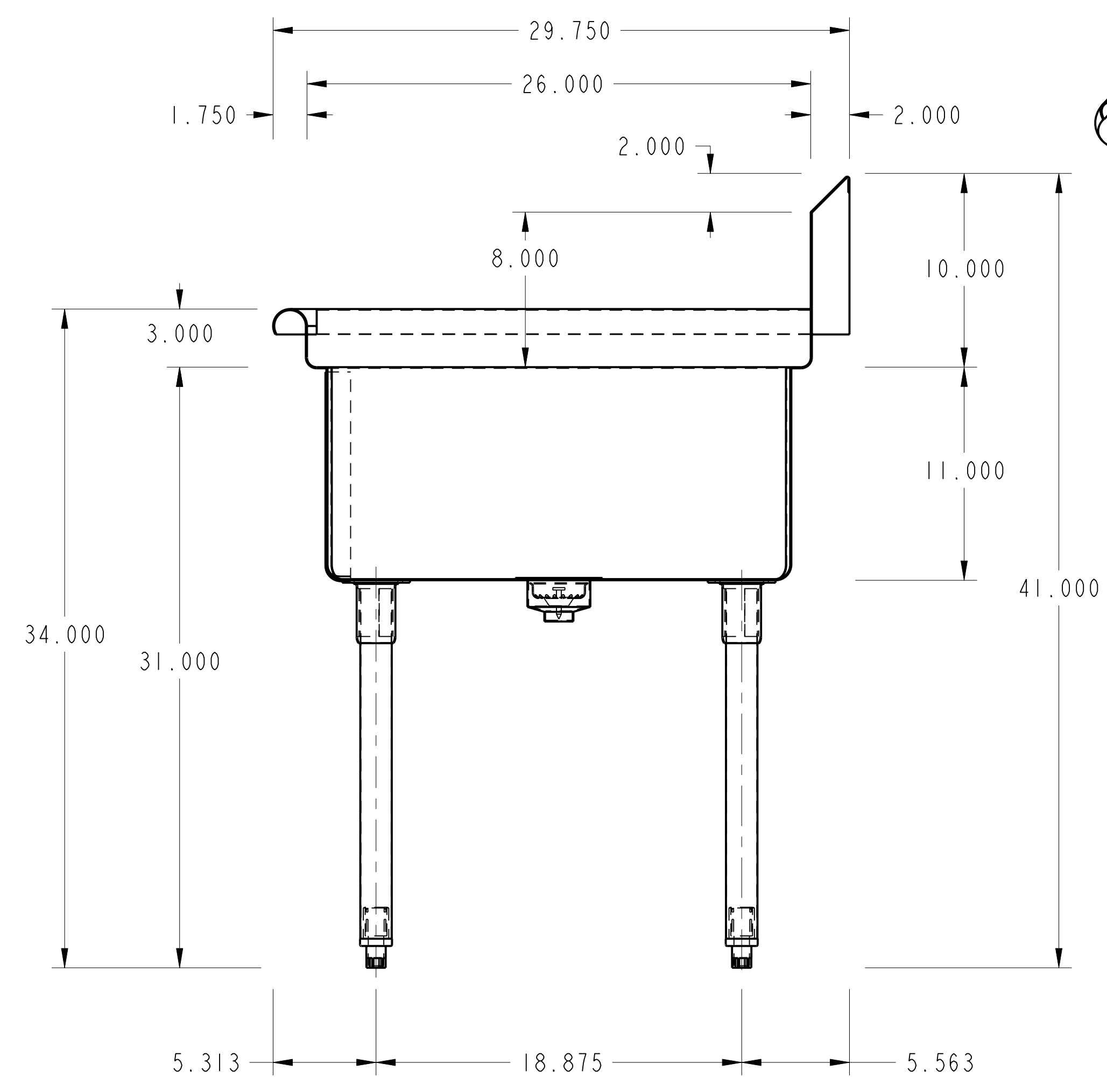
SECTION A-A
