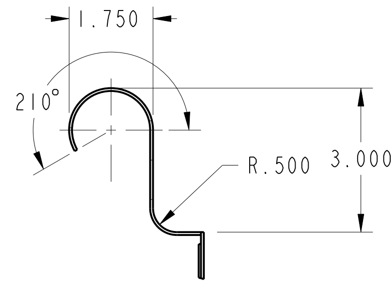
SECTION A-A SCALE 0.500
