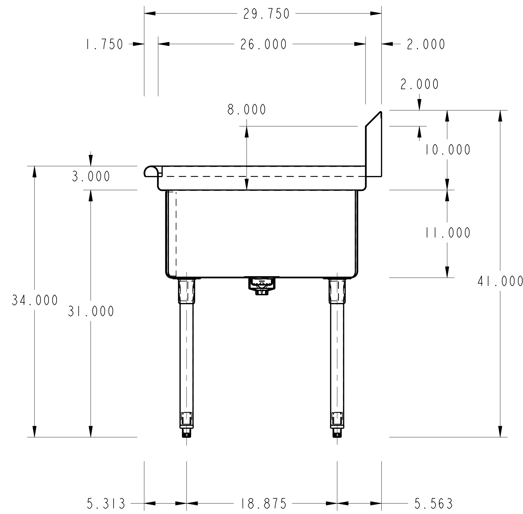
SECTION A-A
