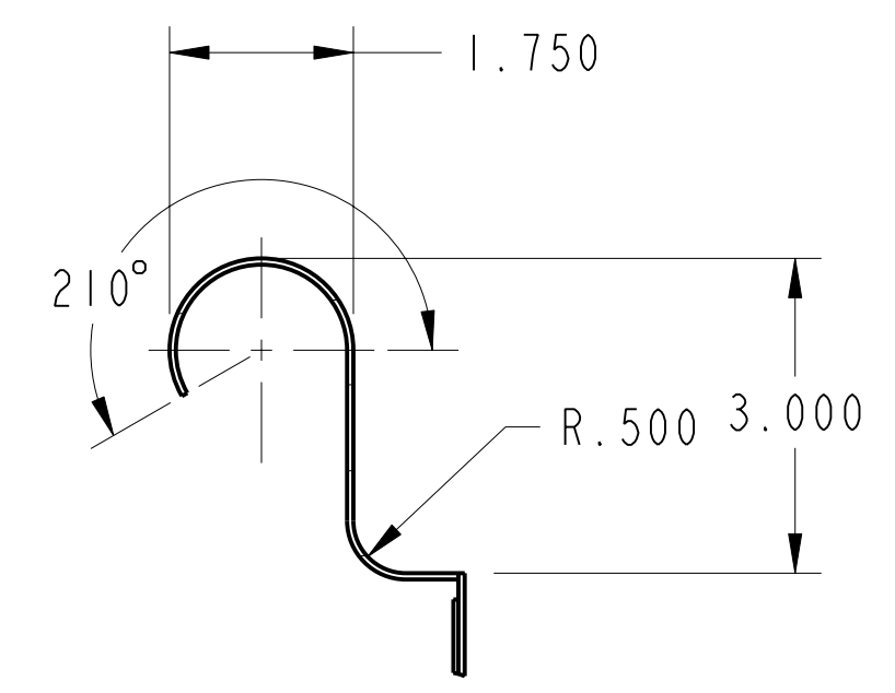
SECTION A-A SCALE 0.500
