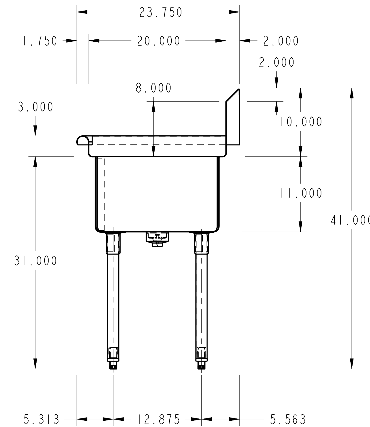
SECTION A-A
