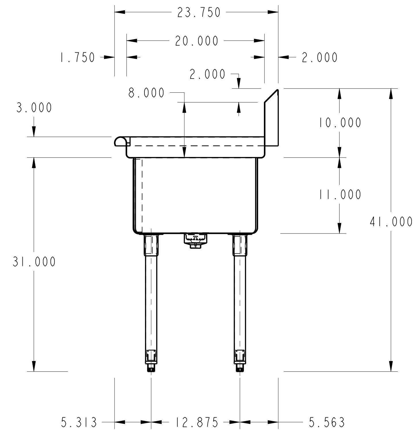
SECTION A-A
