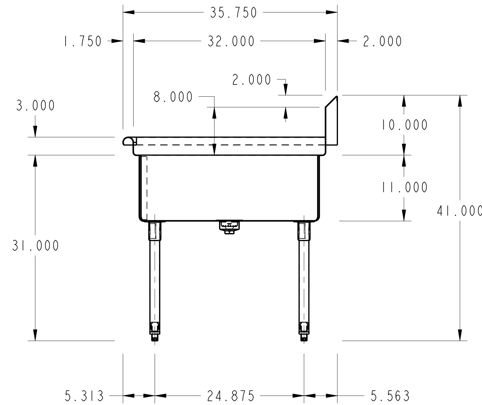
SECTION A-A
