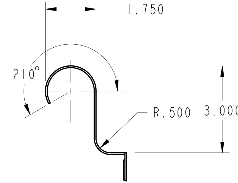
SECTION A-A SCALE 0.500
