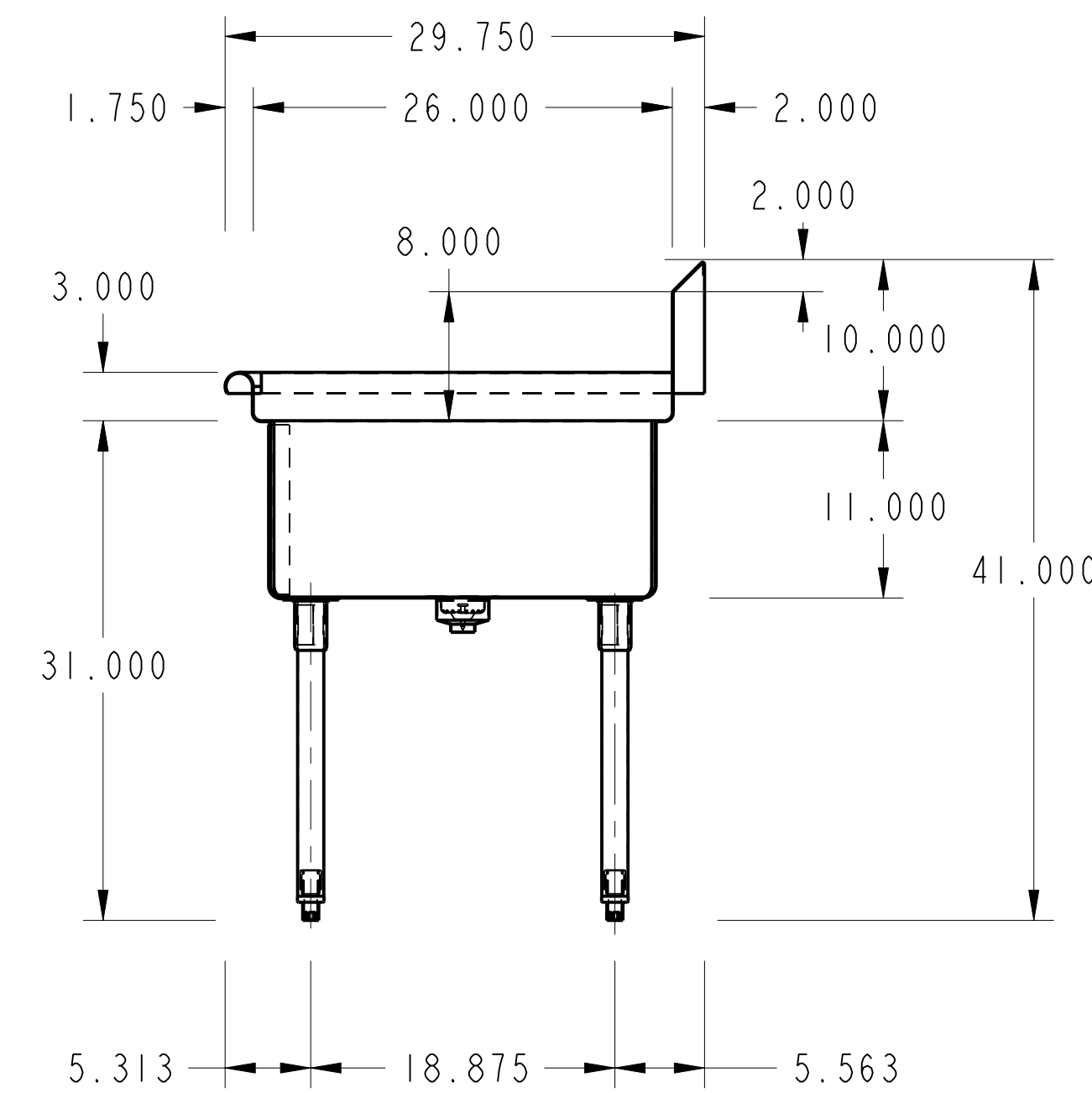
SECTION A-A
