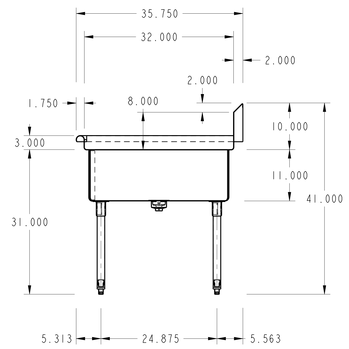
SECTION A-A
