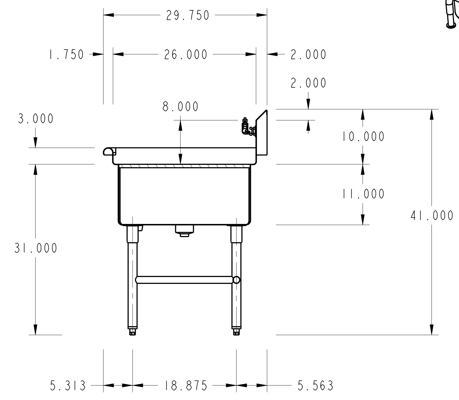
SECTION A-A
