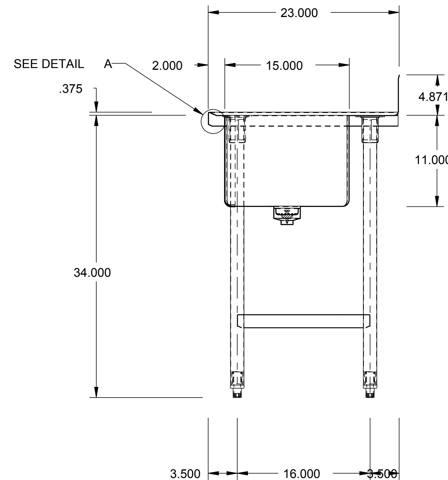
SECTION A-A
