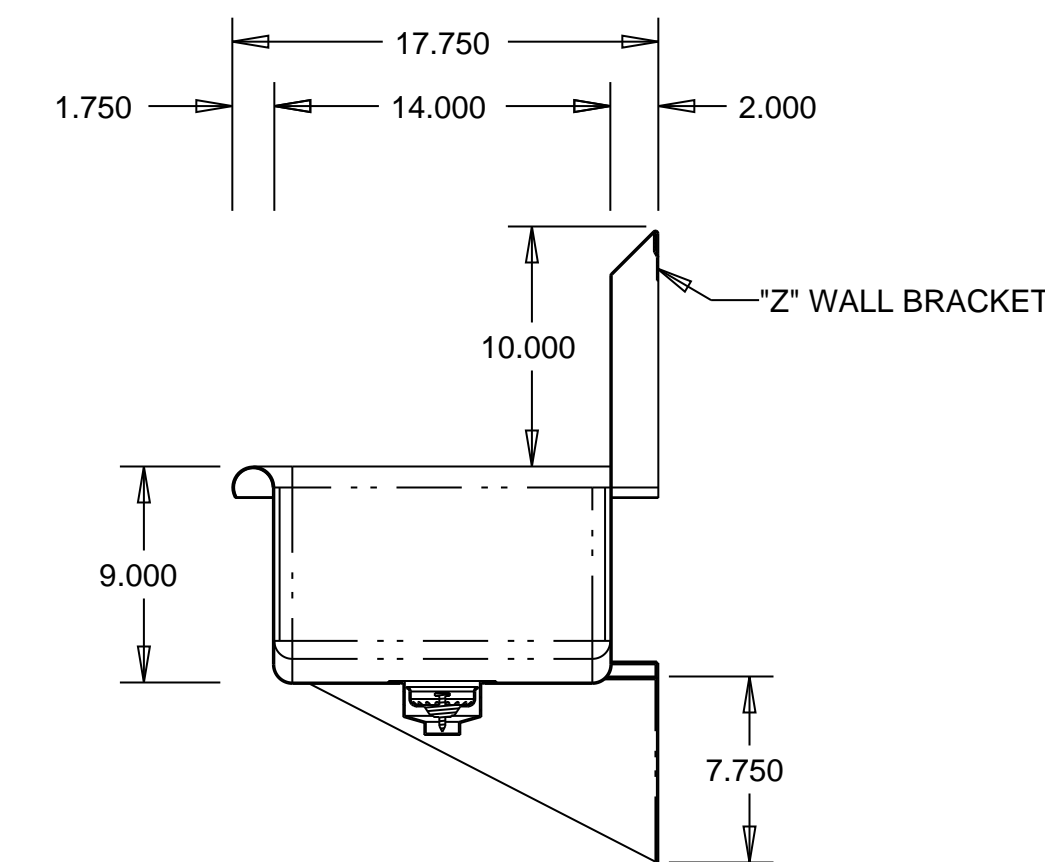
SECTION A-A
