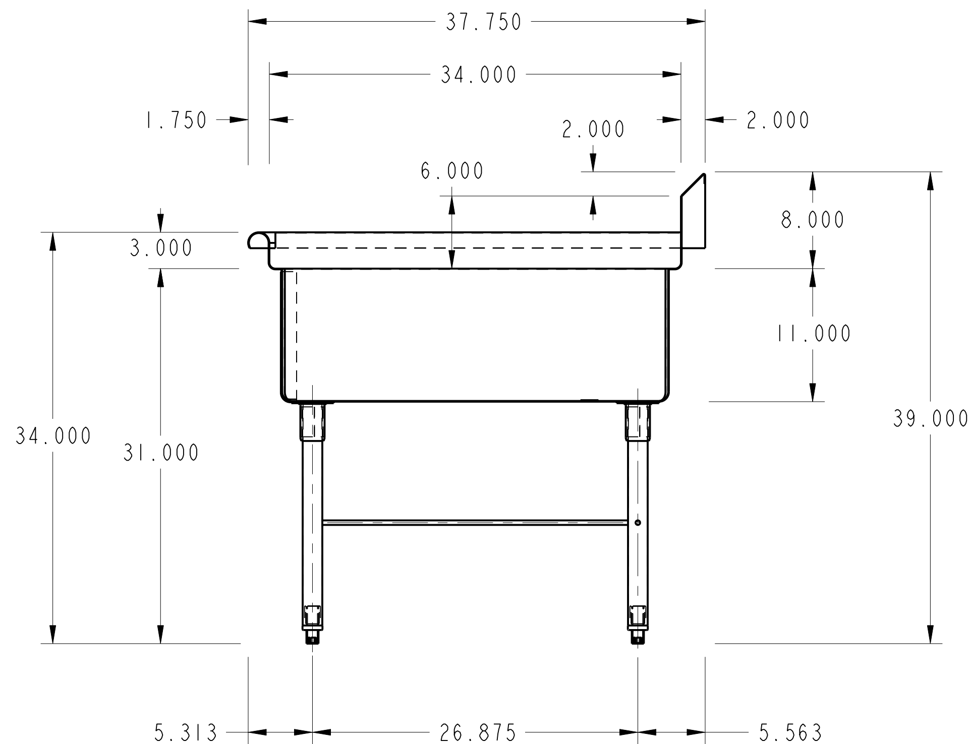
SECTION A-A
